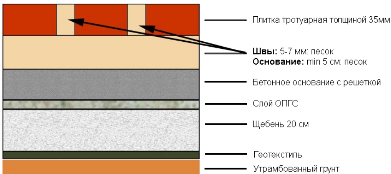
Рис.3. Вариант 3. Значительные нагрузки (заезд тяжелого, крупного автотранспорта)
