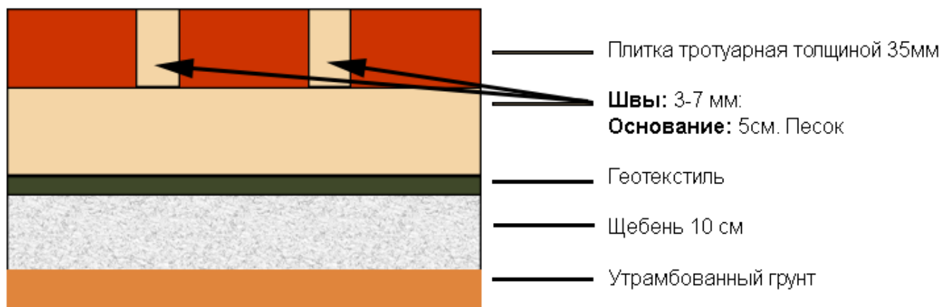
Рис.2. Вариант 2. Средние нагрузки (умеренное движение и стоянка легкового транспорта)
