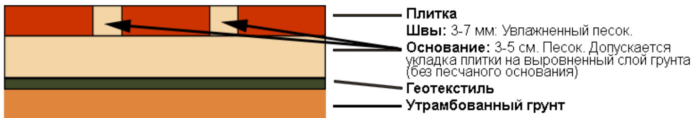
Рис. 1. Вариант 1. Незначительные нагрузки (без заезда автотранспорта)
